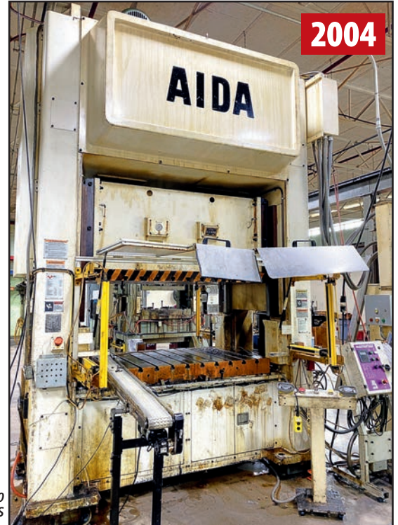
AIDA NSU-S2-200 SSDC PRESS
